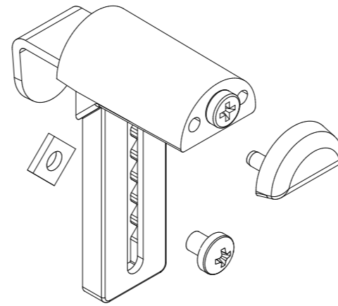
Komponentenansicht
